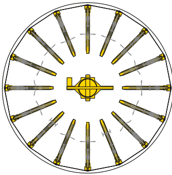
Sezione livello di parcheggio
